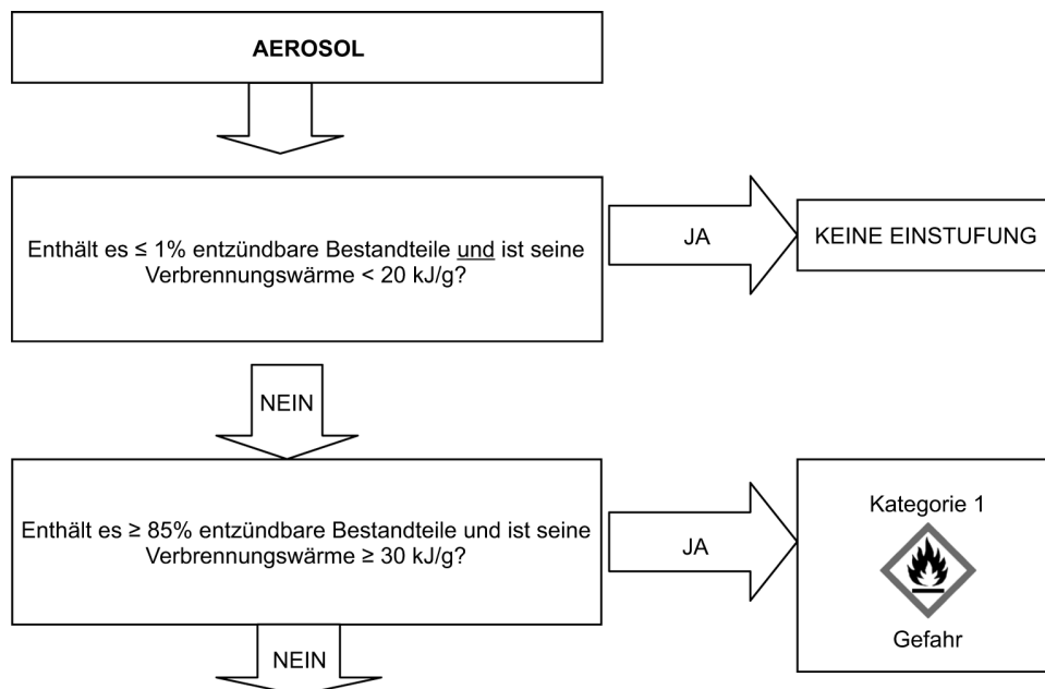
Abbildung 2.3.1 a: entzündbare Aerosole
